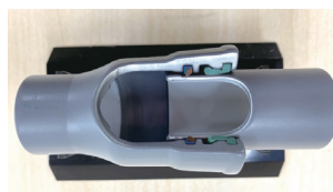
蓮田市で使用している水道管の模型
